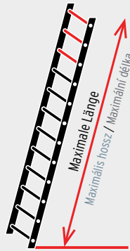
Anlegeleiter Támasztólétra Opěrnéhožebříku
